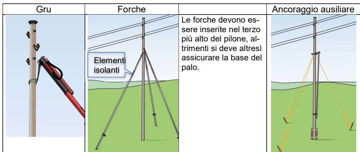
Figura 4 Dispositivi di sicurezza temporanei per il lavoro
