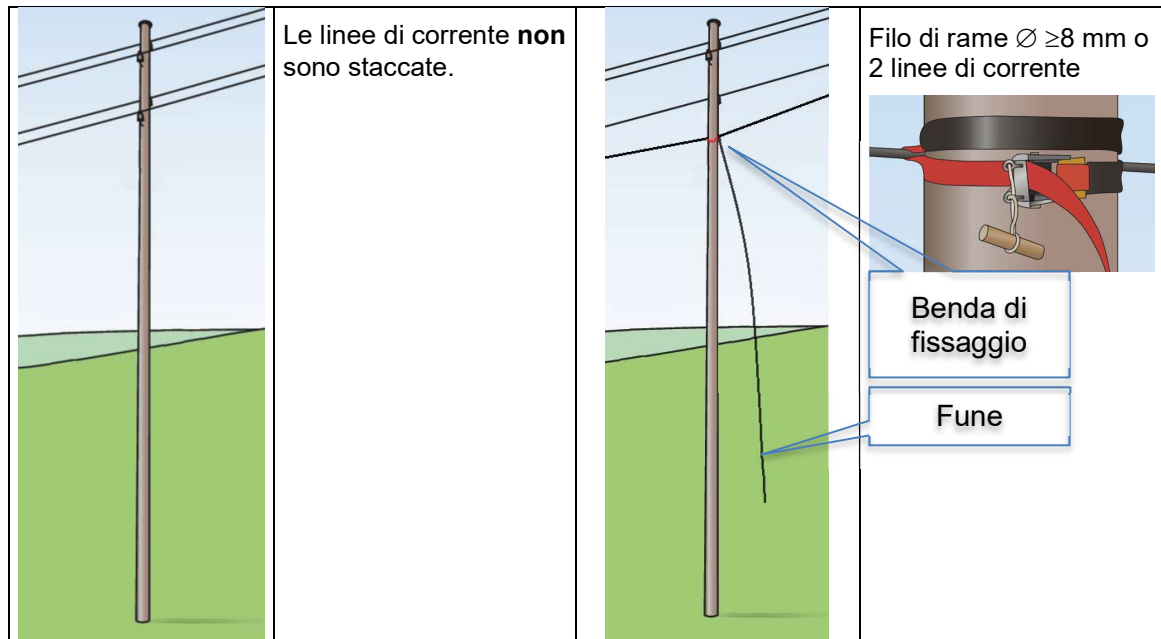
Figura 4 Dispositivi di sicurezza temporanei per il lavoro
