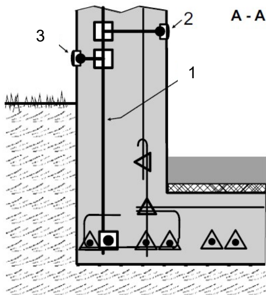
Figura 1c Punti di connessione con protezione EMP
