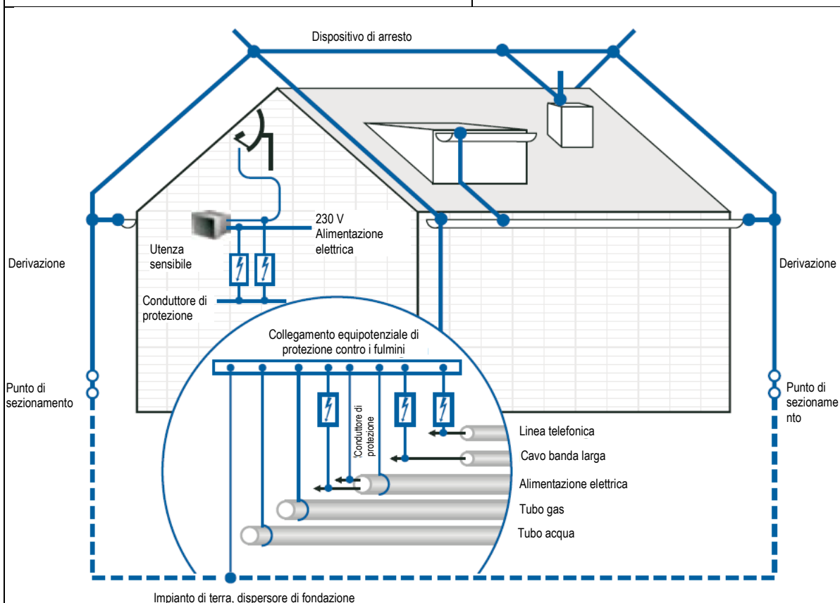
Figura 2: sia la protezione contro i fulmini interna sia quella esterna richiedono controlli regolari da parte di personale opportunamente formato.
