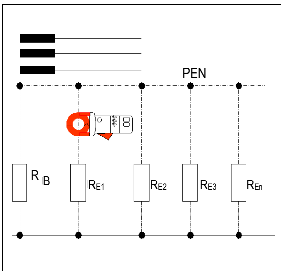
Figura 7: la misurazione, ampiamente diffusa, del loop di messa a terra con una pinza per la verifica della messa a terra non è da sola sufficiente per misurare la resistenza di terra.
