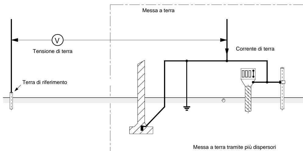
Figura 4: dimensioni della messa a terra secondo l'Ordinanza sulla corrente forte. La tensione misurata tra un dispersore e la terra di riferimento "verso l'esterno" (terreno
