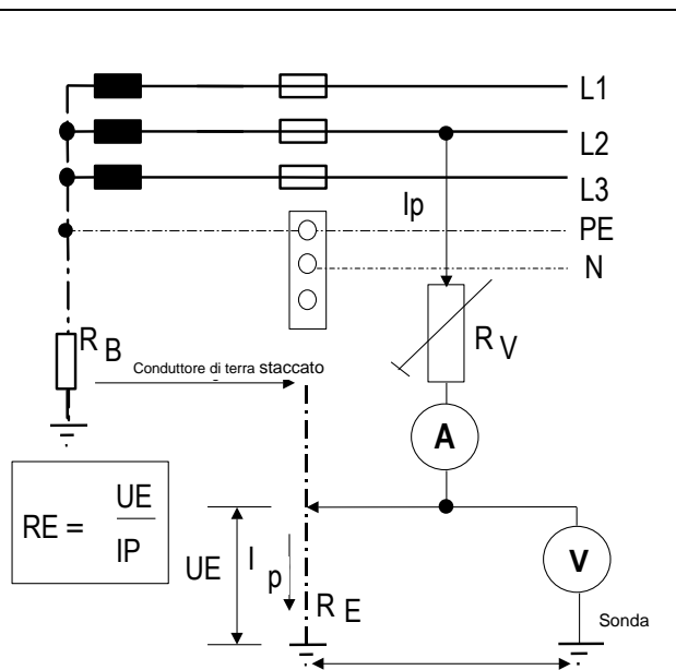
Figura 8: misurazione della messa a terra con l'ausilio della tensione di rete.
