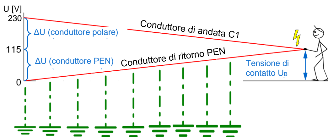
Figura 3: Tensione di contatto
